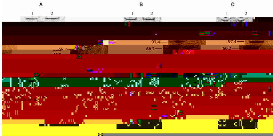
图1 用不同分离胶电泳分离蛋白质标准品的 PAGE
